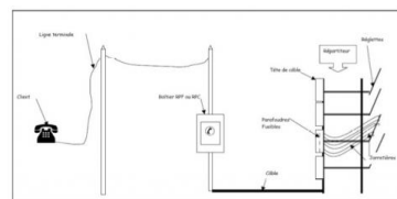
Schéma de disposition des parafoudres radioactifs © DR
